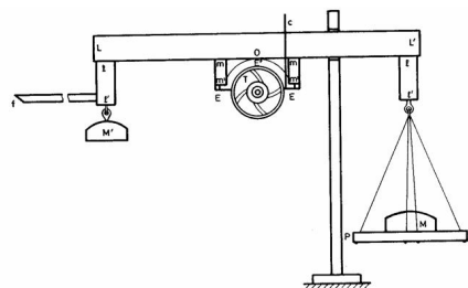
Schéma du dispositif d'essais de Hirn (1862)
